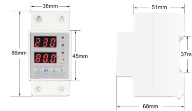
40A/63A/80A dimension
